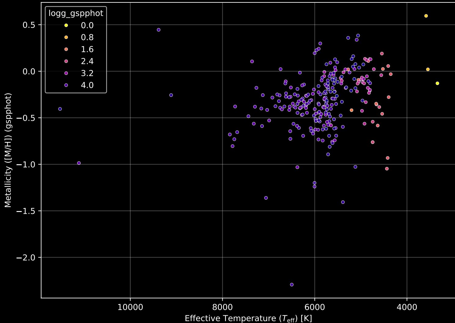
GALAH DR4 Field: [7163] Stellar Population Parameters (n= 264)
