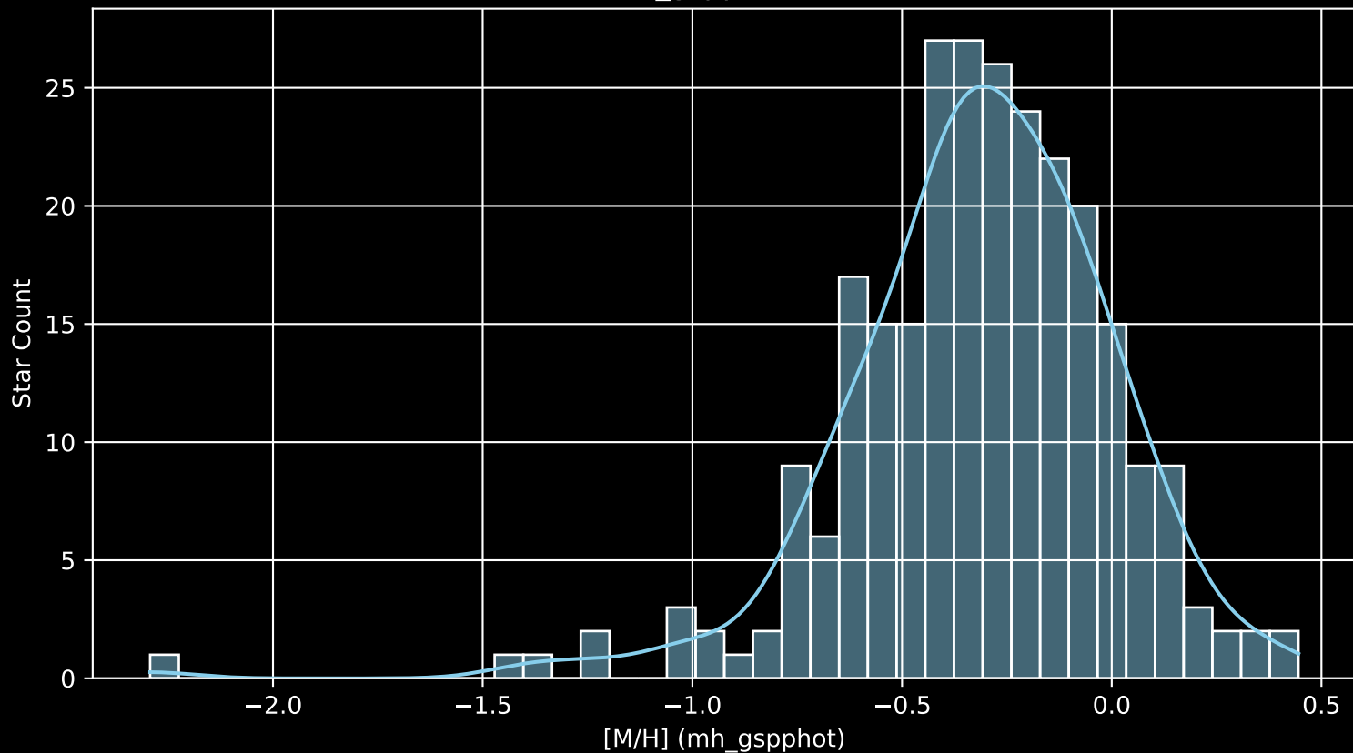
GALAH DR4 Field: [7163] [M/H] (mh_gspphot) (n= 263)
