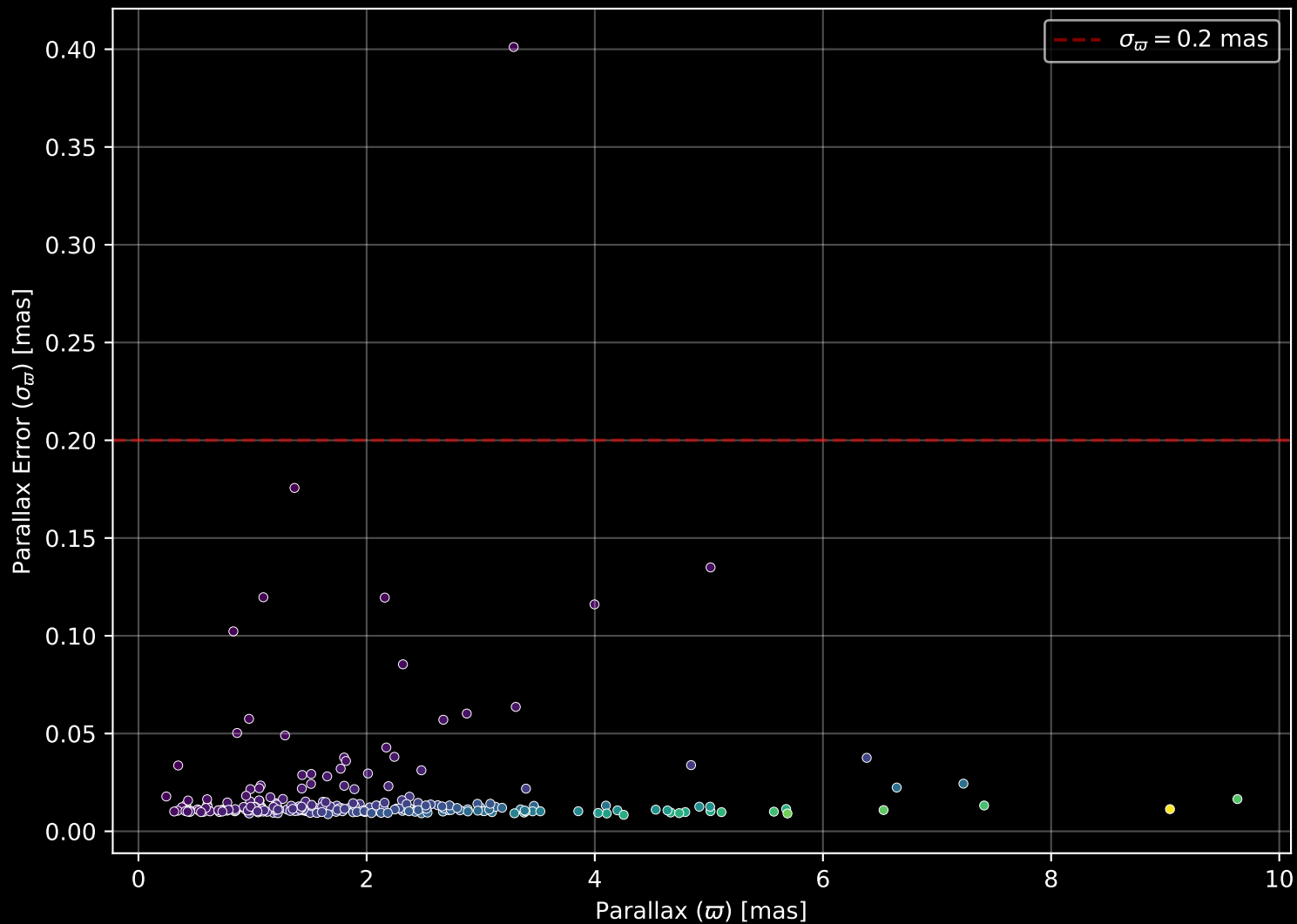
GALAH DR4 Field: [7163] Parallax Quality (n= 264)
