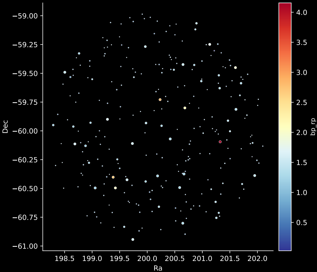
GALAH DR4 Field: [7163] Stars: 264
